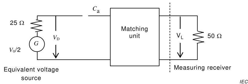
Figure G.7 – Etalonnage de l'antenne monopôle à l'aide de la méthode ECSM
